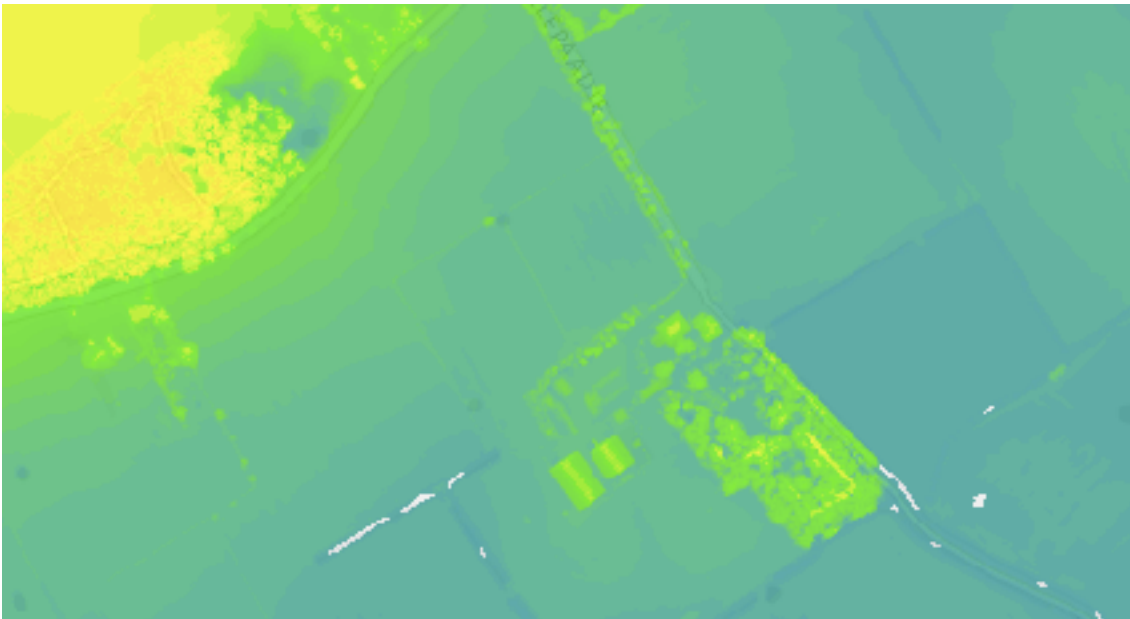
Afb. 4a Detail van het Actueel Hoogtebestand Nederland (AHN2) (2019)
