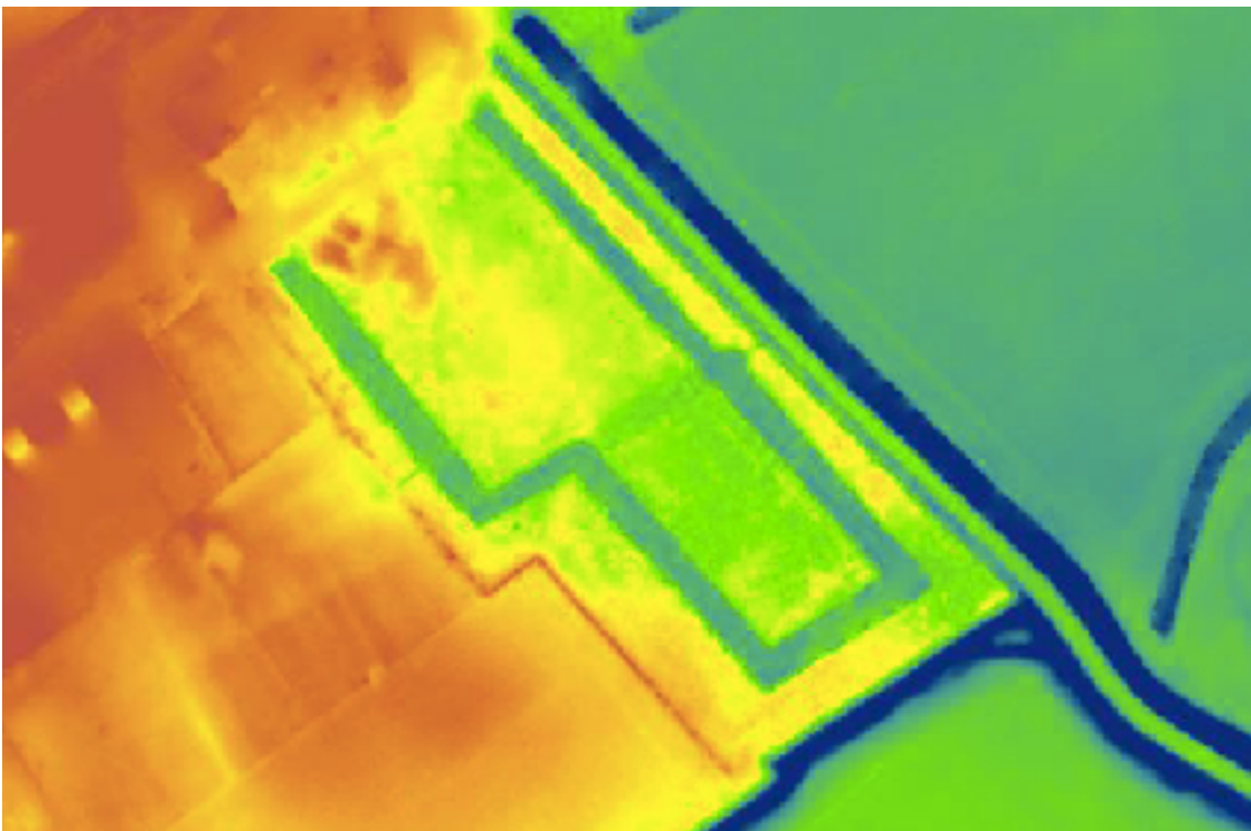
Afb. 4b Detail van de AHN3-kaart, filter: 'maaiveld, blauw, groen, oranje' (2019). Behalve de omgrachting van het huis en de hoger gelegen tuinwal is op deze kaart goed zichtbaar dat de tuin hoger ligt dan het land aan de overzijde van de Skilsloot
