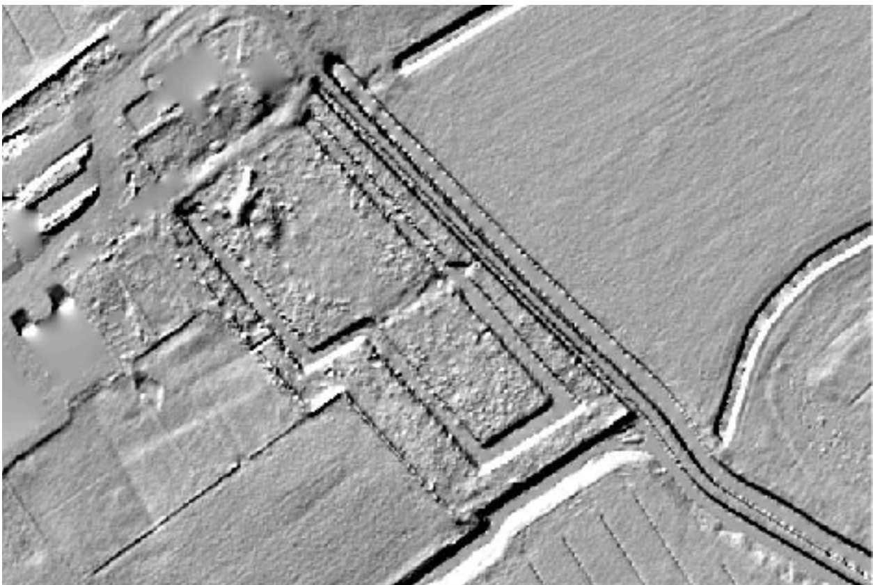
Afb. 4c Algemeen Hoogtebestand Nederland (AHN2), filter: '50 cm maaiveld Hillshade' (2019)
